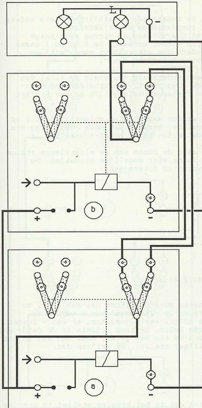
Figuur 4 Hotel-schakeling
